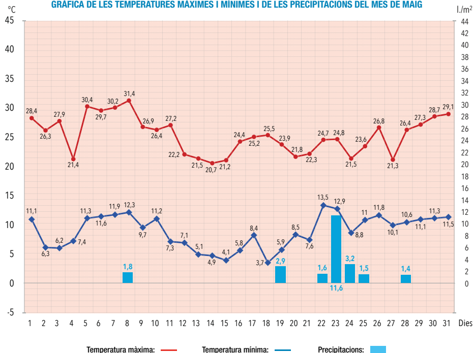
GRÀFICA DE LES TEMPERATURES MÀXIMES I MÍNIMES I DE LES PRECIPITACIONS DEL MES DE MAIG
