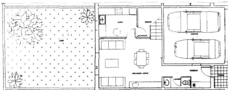
PLANTA BAIXA
