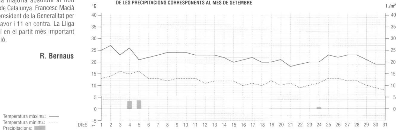
GRÀFICA DE LES TEMPERATURES MÀXIMES I MÍNIMES I DE LES PRECIPITACIONS CORRESPONENTS AL MES DE SETEMBRE
