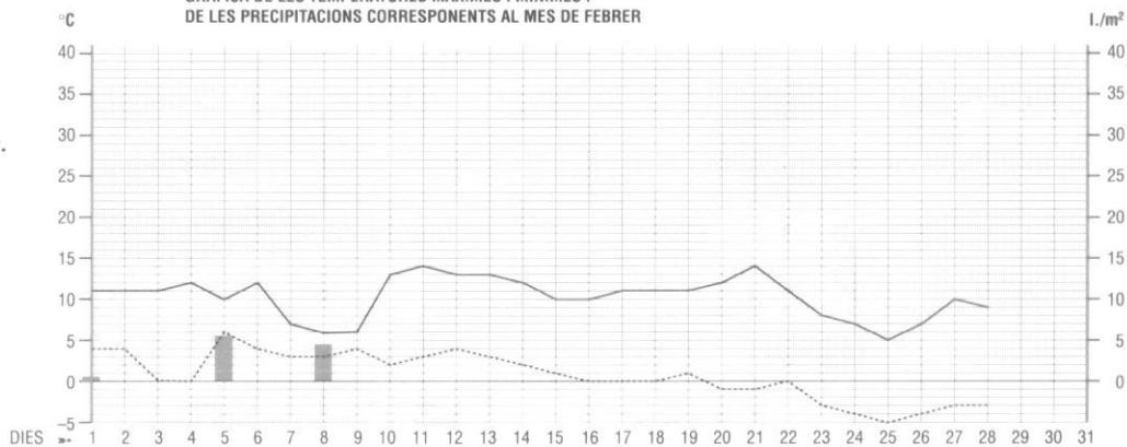
GRÀFICA DE LES TEMPERATURES MÀXIMES I MÍNIMES I DE LES PRECIPITACIONS CORRESPONENTS AL MES DE FEBRER
