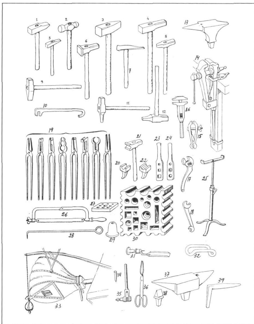
Detall d'eines necessàries per l'ofici de ferrer. 1, 2) martell; 3) mall; 4) escaire mànec fusta; 5) martell petit; 6) plana; 7) martell de pena; 8) tast; 9) tallant; 10) gafa ferrar rodes; 11) punxó; 12) punxó quadrat; 13) enclusa petita; 14) caragol de ferro; 15) caragol de mà; 16, 17, 18) claus; 19) estenalles diferent bucatge; 20) tast d'enclusa (positiu); 21) tast (negatiu); 22) tast d'enclusa (positiu); 23, 24) claveres; 25) mossa; 26) serra; 27) clavera grossa; 28) sirventa; 29) boterola; 30) clavera grossa; 31) botavant; 32) entaulador; 33) manxa; 34) punxó de mà; 35) xitxarra per foradar; 36) estenalles; 37) enclusa; 38) tallant enclusa; 39) tast.
