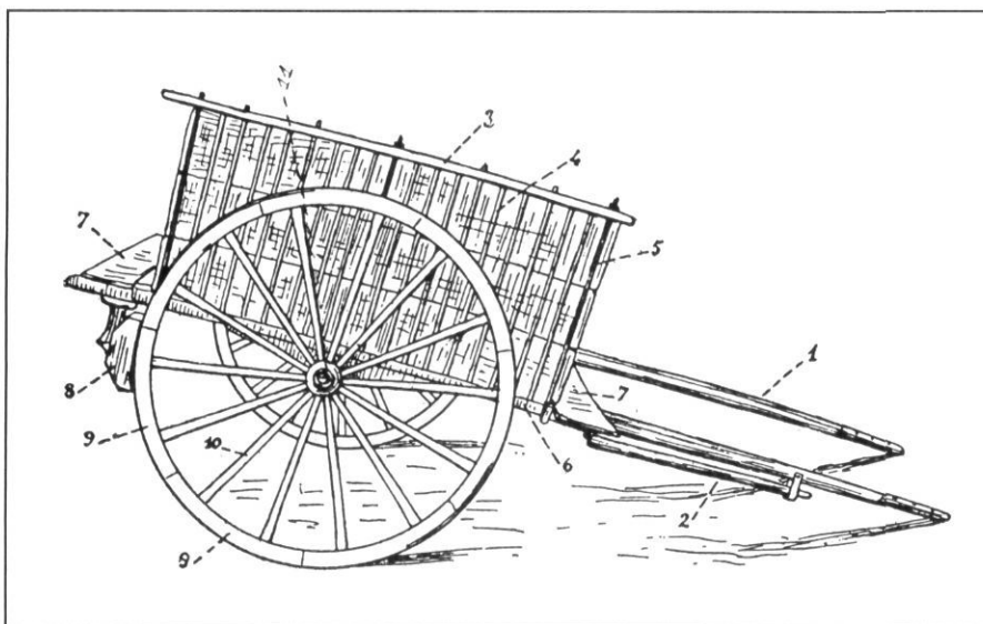
Carro d'escala. 1) braç; 2) descans; 3) barana; 4) empostats costat; 5) empostats davant; 6) contraperna; 7) tablilla; 8) soc; 9) corba; 10) raig; 11) botó. (Dicc. Alcover-Moll)
