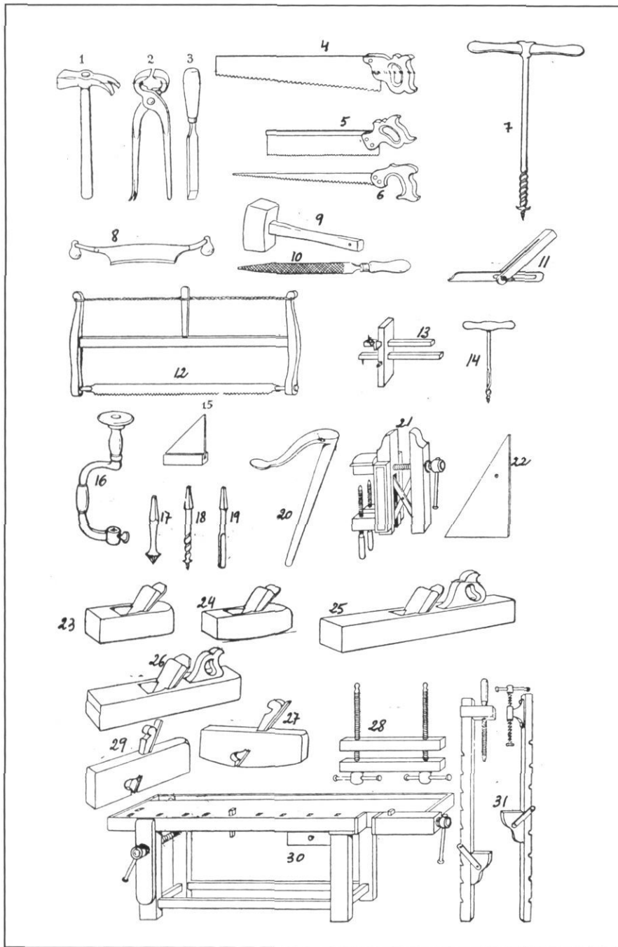
Detall d'eines necessàries per l'ofici de carreter. 1) martell; 2) estenalles; 3) enformador; 4) xerrac de mà; 5) xerrac beina; 6) xerrac de punta; 7) barrina; 8) cantell; 9) maça de fusta; 10) raspa; 11) sentenella; 12) serra; 13) rosset; 14) barrina; 15) cartabó; 16) filaberquí; 17, 18, 19) broques; 20) batlet; 21) caragol de ferro; 22) escaire; 23) ribot pla; 24) ribot corbat; 25) garlopa; 26) garbopí; 27) guillaume corbat; 28) congrells; 29) guillaume; 30) banc de fusta; 31) allicador.
