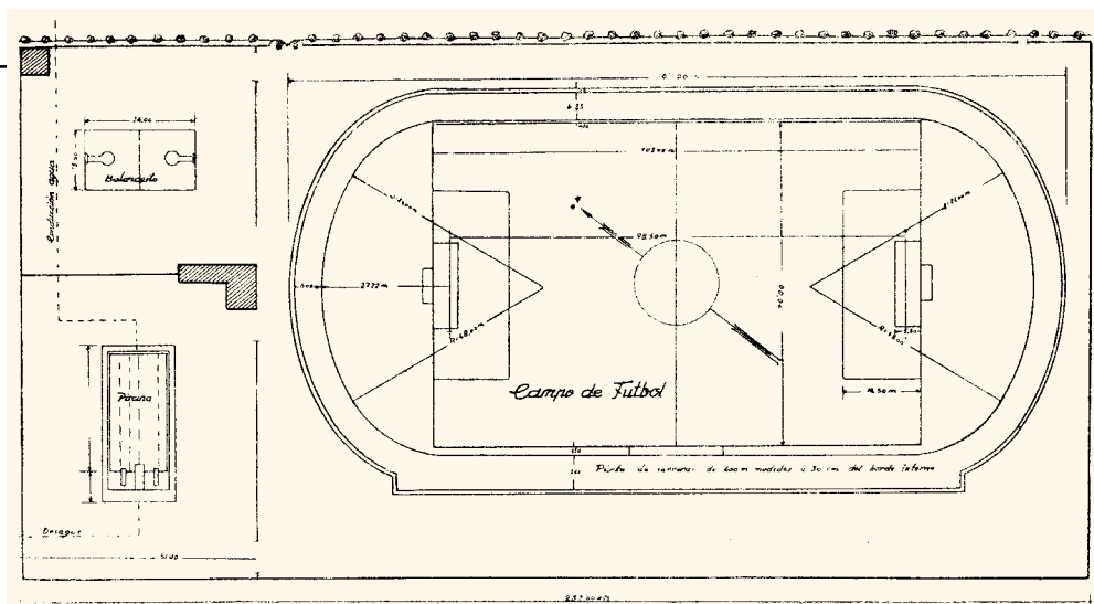
Esquema i dimensions de les instal·lacions publicat al programa de la Festa Major d'aquell any.
