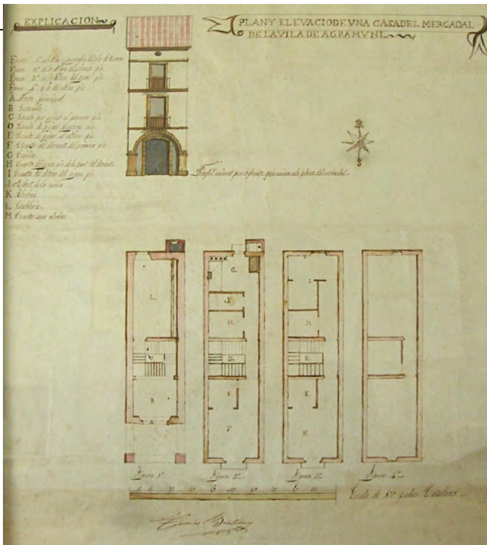
Alçat i planta d'una casa del Mercadal, signat per Tomàs Bertran el 1804.
