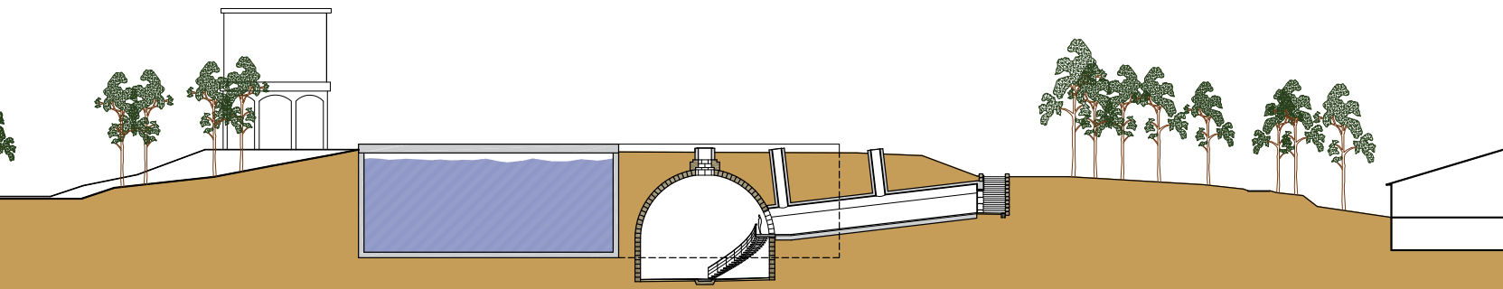
Secció del plànol de l'accés a la Cisterna del Convent dels Franciscans que antigament hi havia al cim del tossal on es van instal·lar els primers dipòsits de distribució d'aigua.
