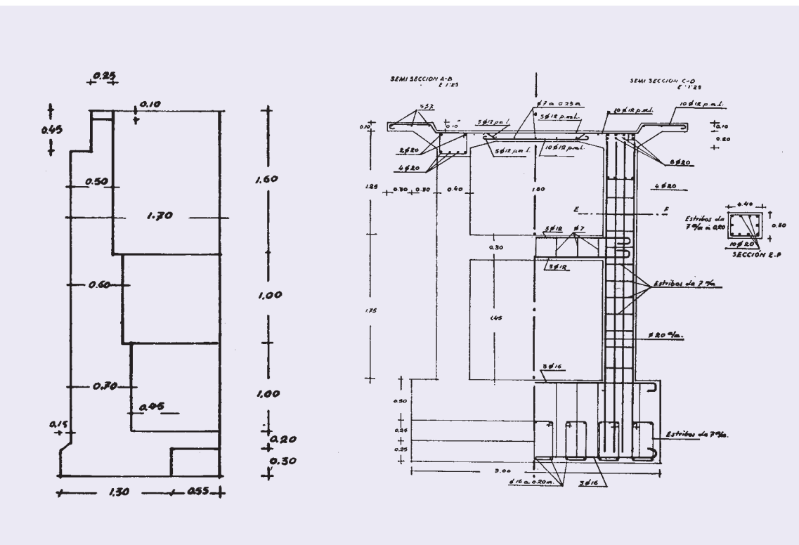
Tres imatges amb els seus esquemes del nou pont que es va construir per donar servitud de pas als horts de les Planes.
