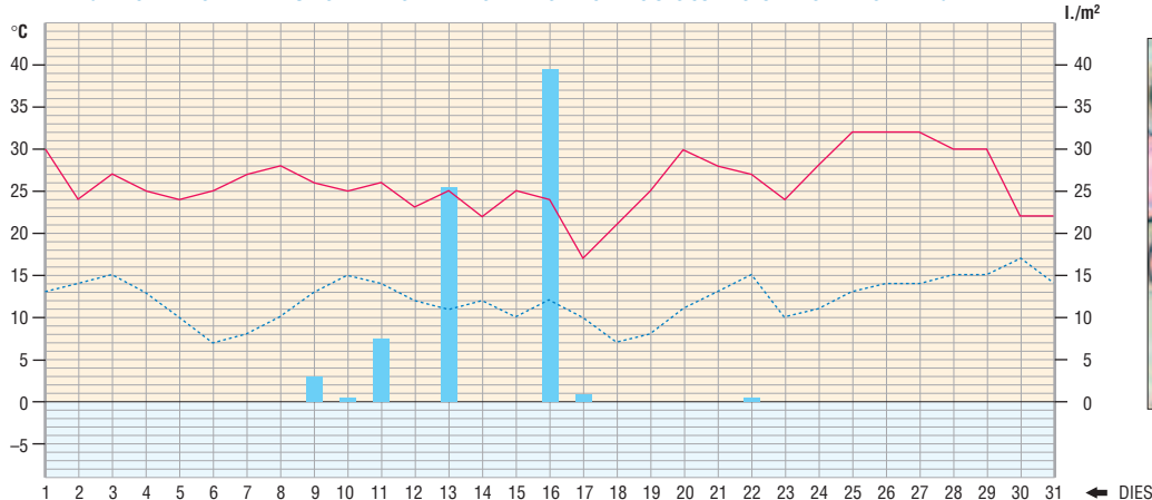
GRÀFICA DE LES TEMPERATURES MÀXIMES I MÍNIMES I DE LES PRECIPITACIONS CORRESPONDENTS AL MES DE MAIG
