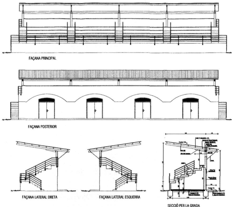
Plànol de la nova construcció de les grades del camp de futbol.
