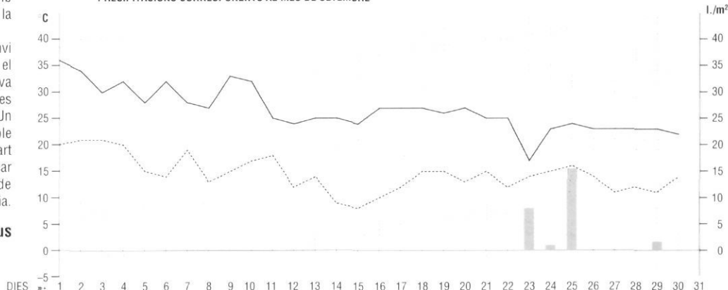
GRÀFICA DE LES TEMPERATURES MÀXIMES I MÍNIMES I DE LES PRECIPITACIONS CORRESPONENTS AL MES DE SETEMBRE
