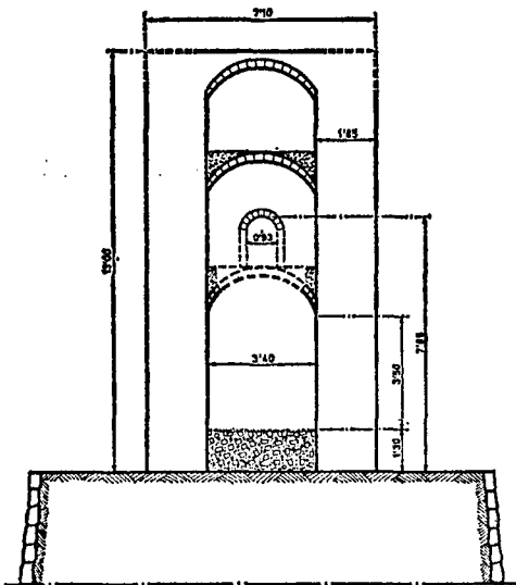
SECCIO TORRE D'ALMENARA
