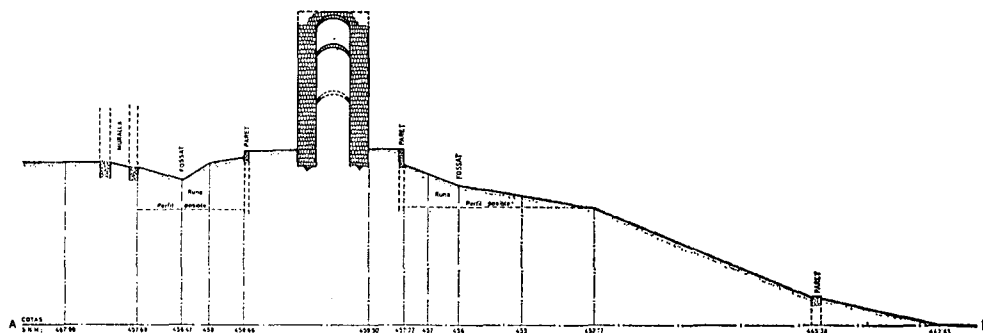
PERFIL TORRE D'ALMENARA I TERRENY
